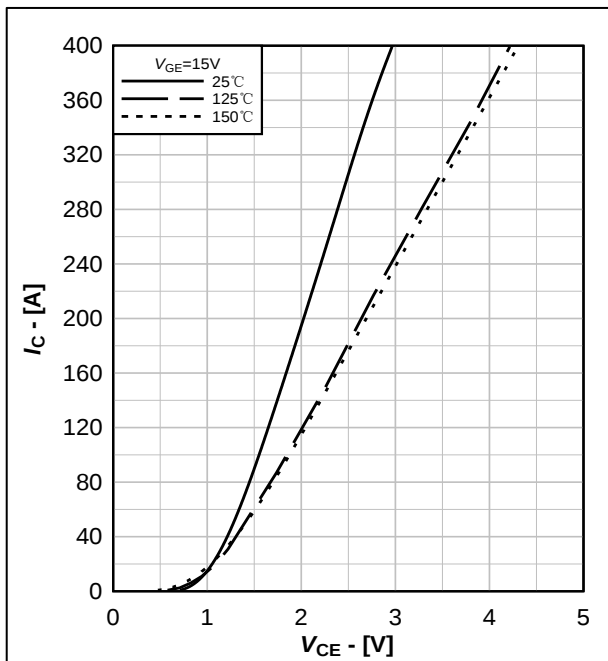
图 5. IGBT 输出特性典型曲线, I_C = f(V_{CE})
