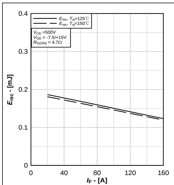
图 19. FRD 反向恢复损耗典型曲线, E_{rec}=f(I_F)
