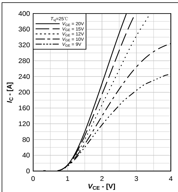
图 3. IGBT 输出特性典型曲线, I_C = f(V_{CE})
