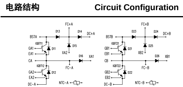
图 1. 电路结构 Fig. 1 Circuit configuration
