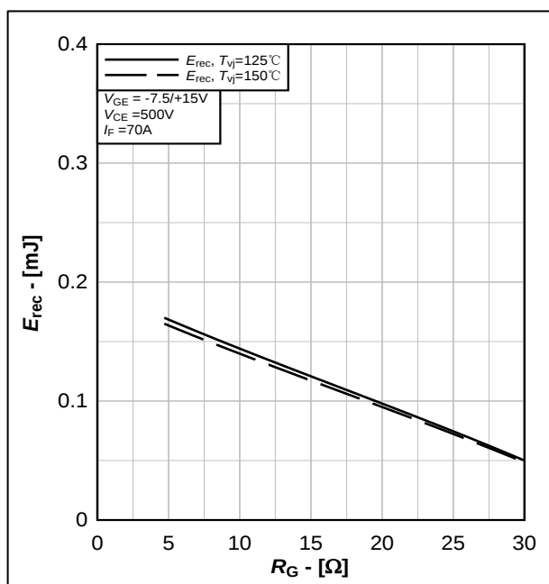
图 20. FRD 反向恢复损耗典型曲线, E_{rec}=f(R_G)
