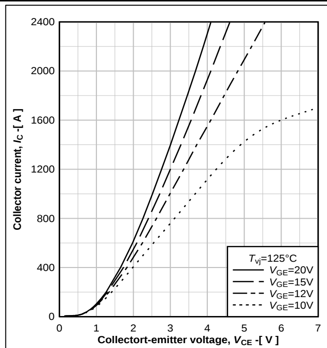
图4. 输出特性典型曲线
