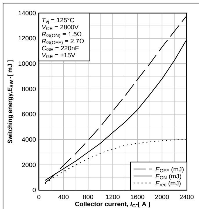
图5. 开关能耗与集电极电流关系曲线
