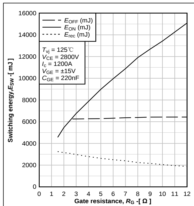
图6. 开关能耗与栅极电阻的关系曲线
