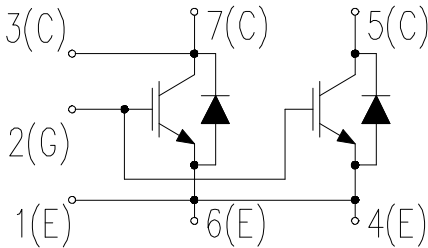
图 1.电路结构 Fig. 1 Circuit configuration
