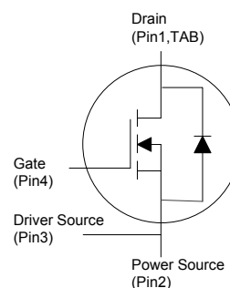
图 1. 电路结构
