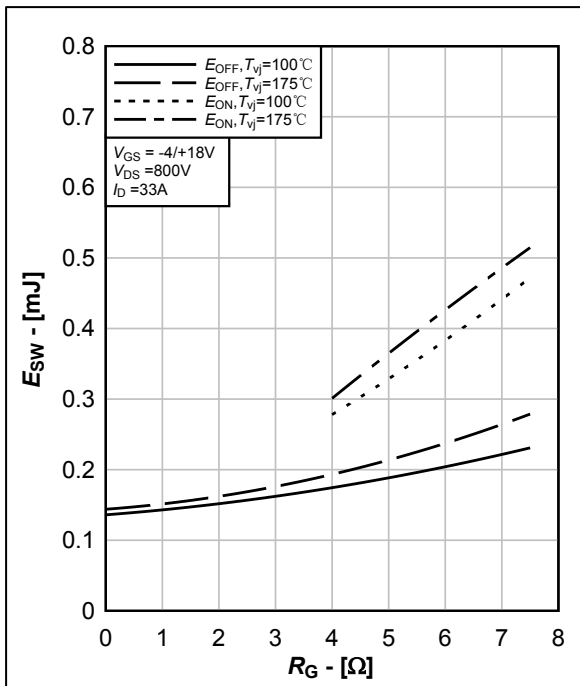
图 11. MOSFET 开关损耗典型曲线, E_{on}=f(R_G) , E_{off}=f(R_G)
