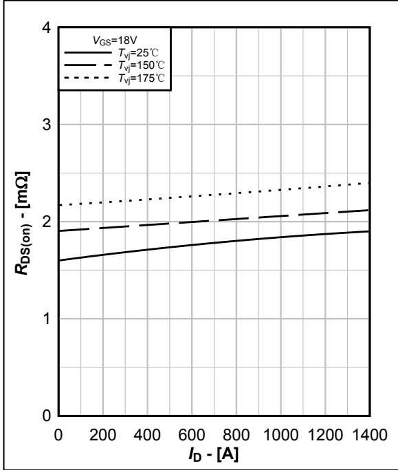
图 7. 导电电阻典型曲线, R_{DS(on)} = f(I_D)
