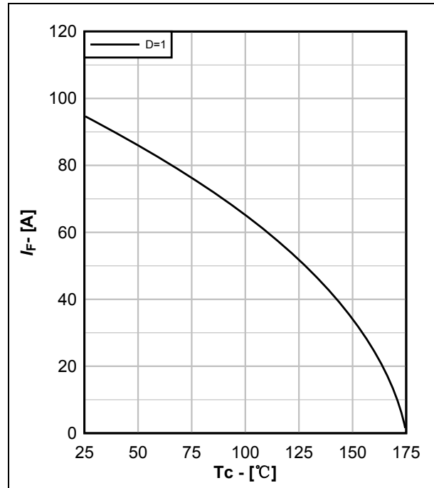
图 3. 不同负载下的电流曲线, I_F = f(T_c)
