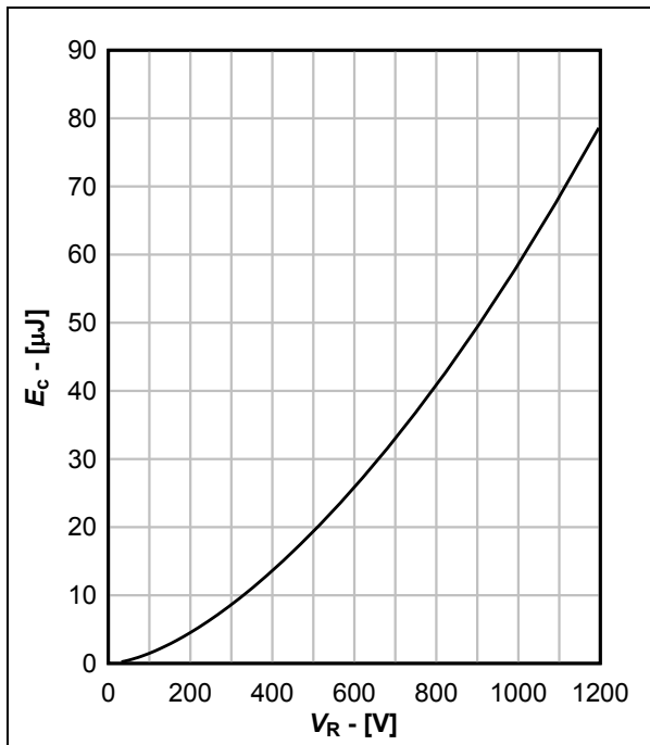
图 8. 典型电容能量与反向电压曲线, E_C = f(V_R)
