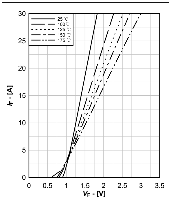
图 4. 典型正向特性曲线, I_F=f(V_F)
