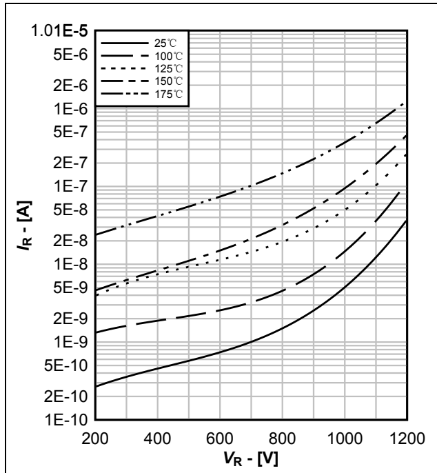
图 6. 典型反向特性曲线, I_R = f(V_R)
