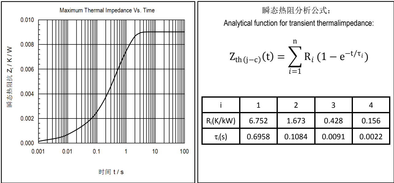
图2. 瞬态热阻抗曲线及分析公式
