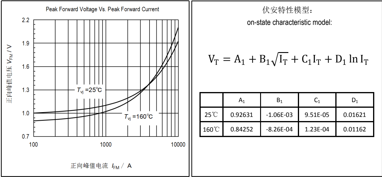
图1. 正向伏安特性曲线及拟合公式
