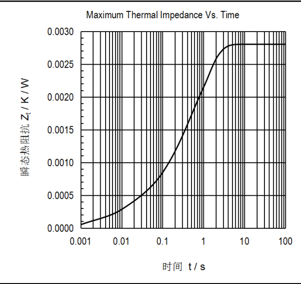
图2. 瞬态热阻抗曲线及分析公式
