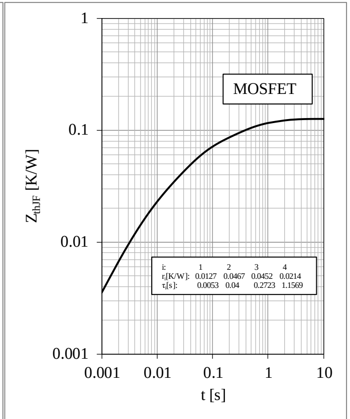
Fig 10. MOSFET Transient Thermal Impedance
