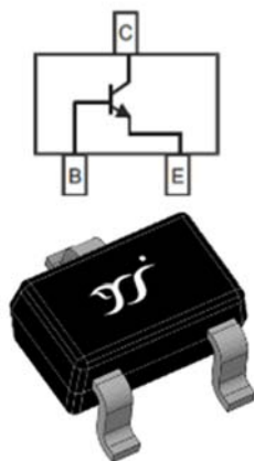
SOT-323
