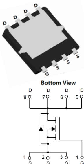
PDFN5060-8L
